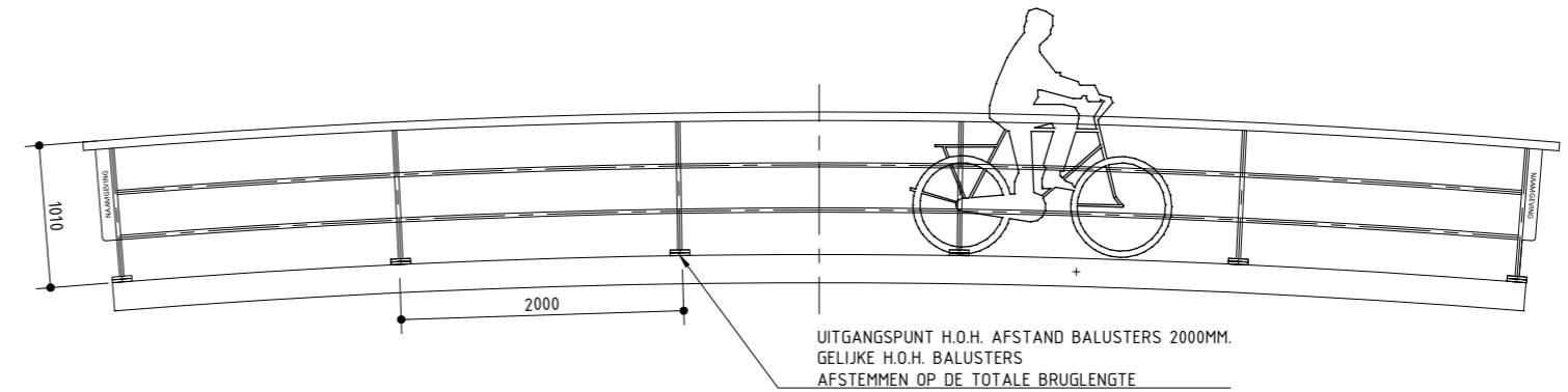
HEKWERK TYPE LANDELIJK
