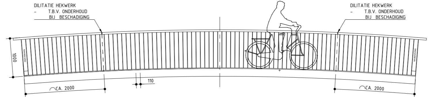
HEKWERK TYPE STEDELIJK
