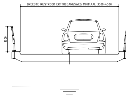
5. VERKEERSBRUG ZONDER VOETGANGERSSTROOK
