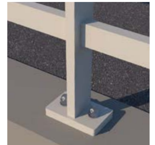
DETAIL VOETPLAAT
