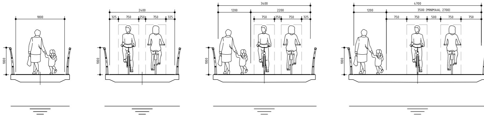
1. VOETGANGERSBRUG 2. VOETGANGERS-, FIETSBRUG 3. VOETGANGERS-, FIETSBRUG MET LOSSE VOETGANGERSSTROOK 4. VOETGANGERS-, FIETSBRUG MET LOSSE VOETGANGERSSTROOK, HOGE INTENSITEIT
