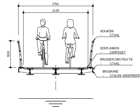
VOORBEELD DOORSNEDEN BRUGDEKCONSTRUCTIE - STAAL
