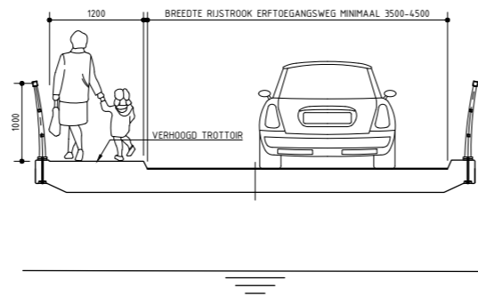
6. VERKEERSBRUG MET VOETGANGERSSTROOK
