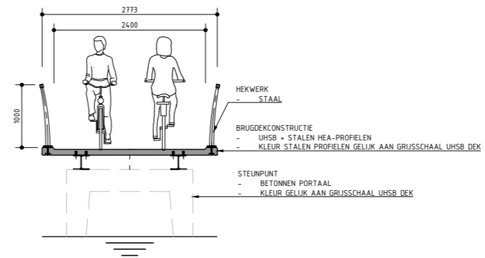
VOORBEELD DOORSNEDEN BRUGDEKCONSTRUCTIE - UHSB + STALEN LIGGERS
