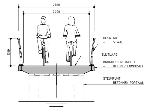
VOORBEELD DOORSNEDEN BRUGDEKCONSTRUCTIE - BETON OF COMPOSIEET
