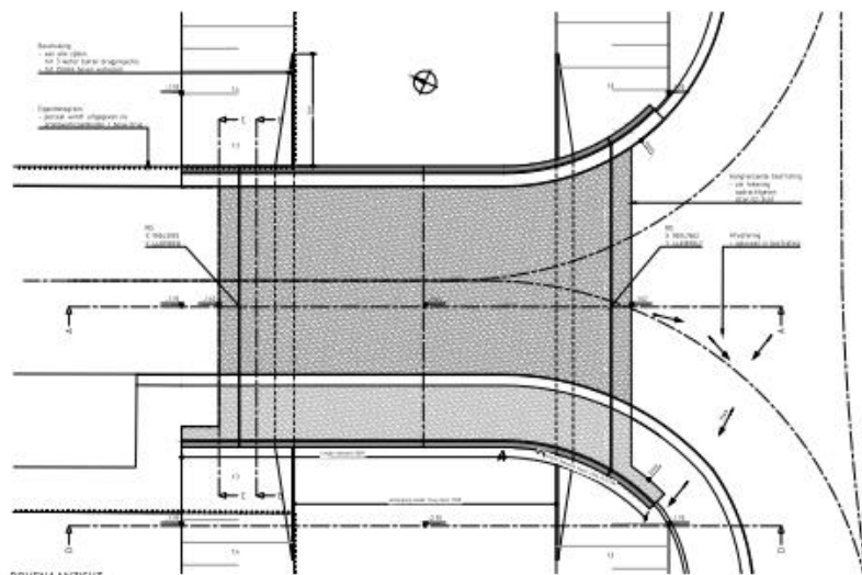
BOVENAANZICHT
