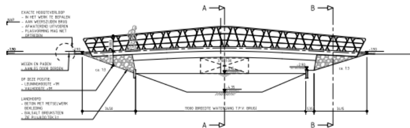
ZIJAAANZICHT SCHAL 100
