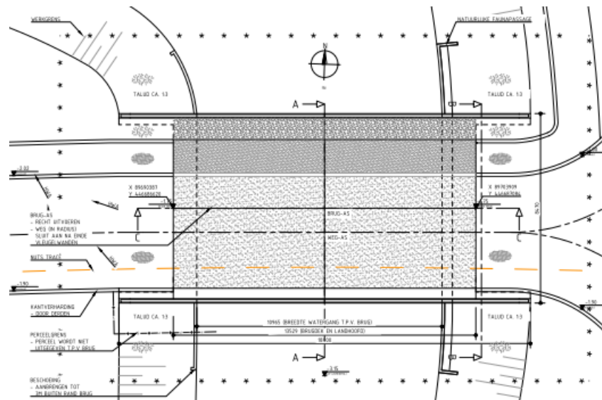
BOVENAANZICHT SCHAL 100
