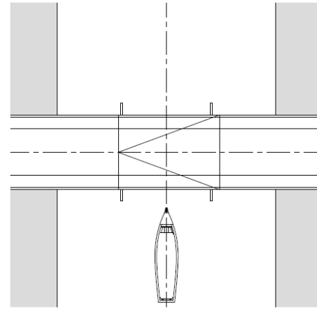
afb. 31 - klapbrug
