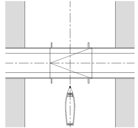
afb. 32 - ophaalbrug
