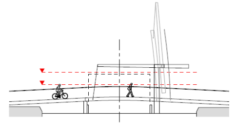
afb. 32 - ophaalbrug
