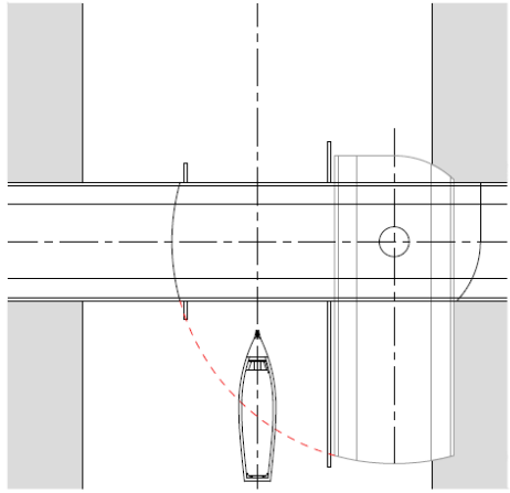
afb. 28 - draaibrug
